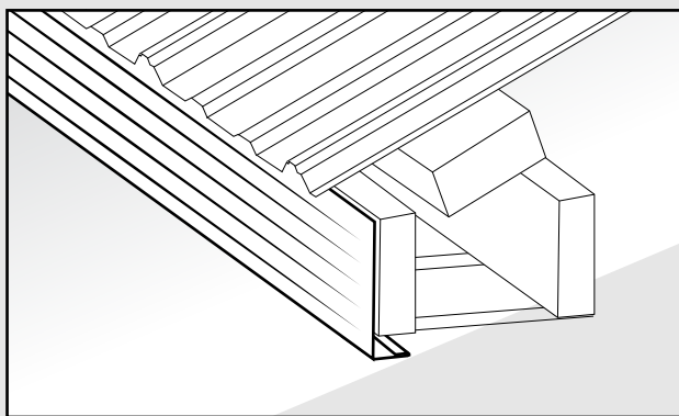
Fascia Trim
