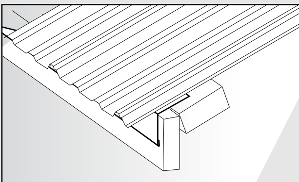
Drip Edge
